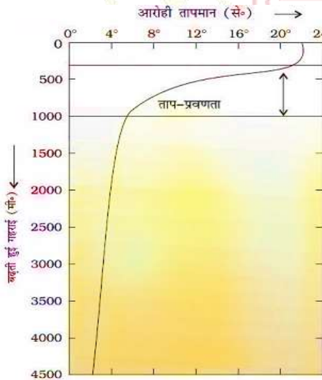
चित्र- 4.3 ताप प्रवणता
