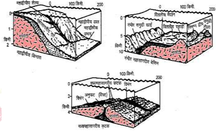
चित्र-4.2 महासागरीय अधस्तल के उच्चावच
