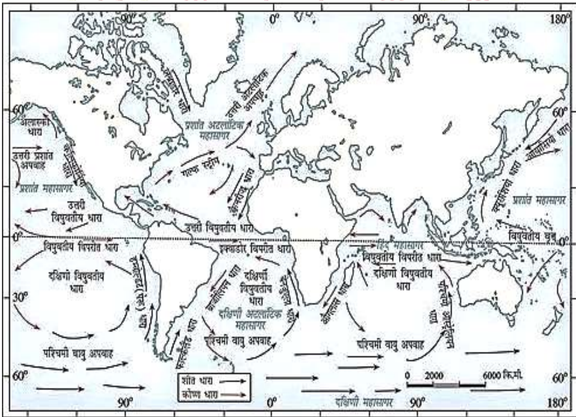
चित्र- 4.5 महासागरीय धाराएँ
