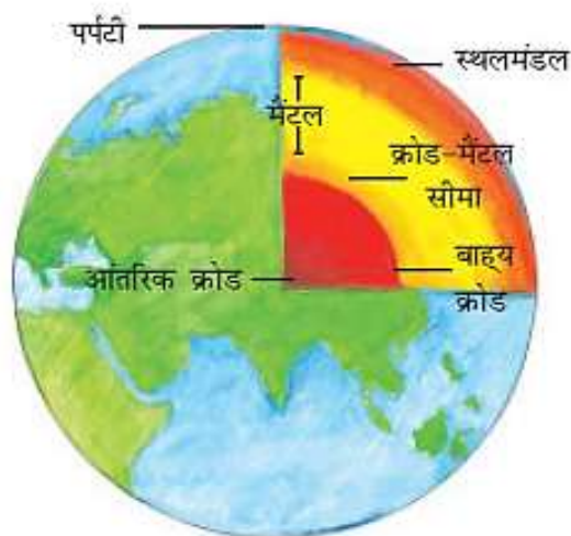
चित्र 2.1- पृथिवी की आन्तरिक संरचना
