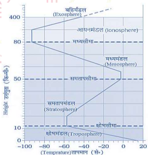
चित्र-3.1 वायुमण्डल की संरचना
