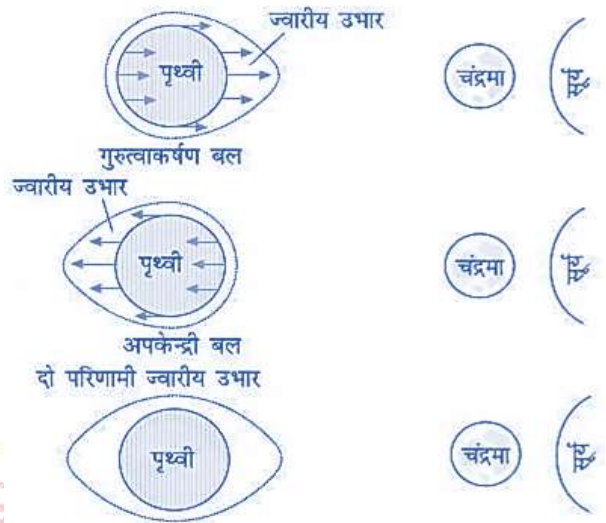
चित्र-4.4 गुरुत्वाकर्षण बल और ज्वार भाटा के मध्य
